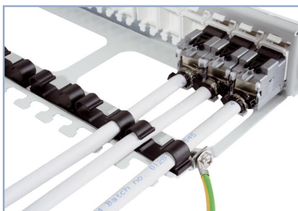
Câblage arrière non figé, assuré par les clips de la série FLEX
