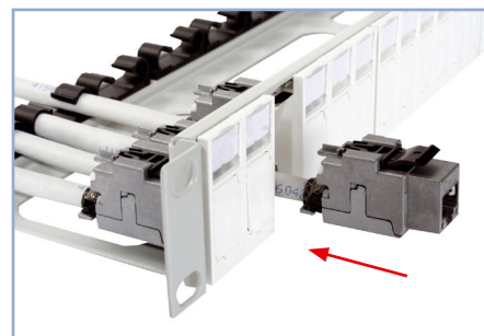
Câblage et montage par la face avant
