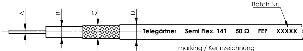
marking / Kennzeichnung
