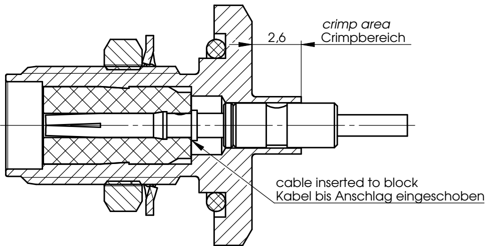
crimp insert / Crimpeinsatz: N01001A0010
